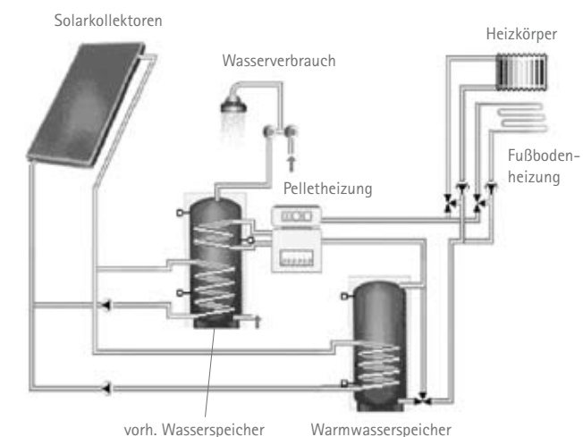
Schematische Darstellung eines möglichen Energieverbundes
